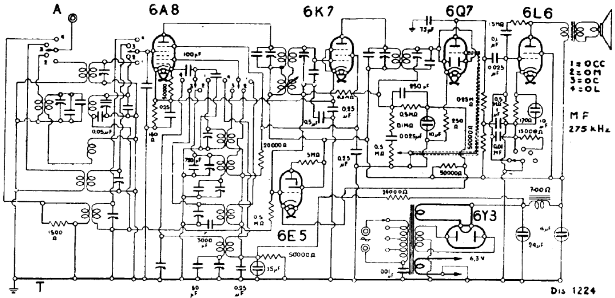
IRRADIO - MOD. « D X 7 »
